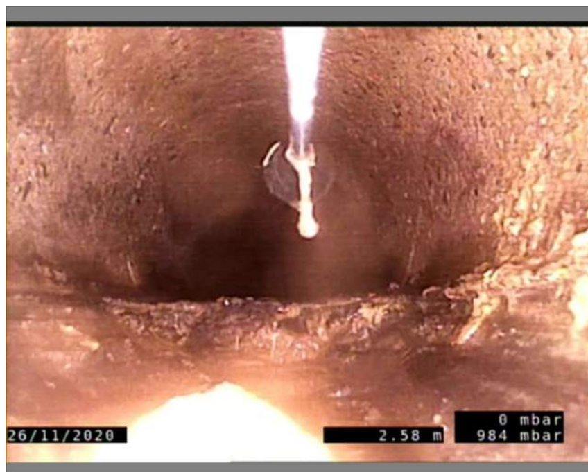
Foto: BR2-BR3-261120-2,58-3-A.JPG 2,58m, Aflejring klasse 3, fra urref 4 til urref 8, Fastsiddende
