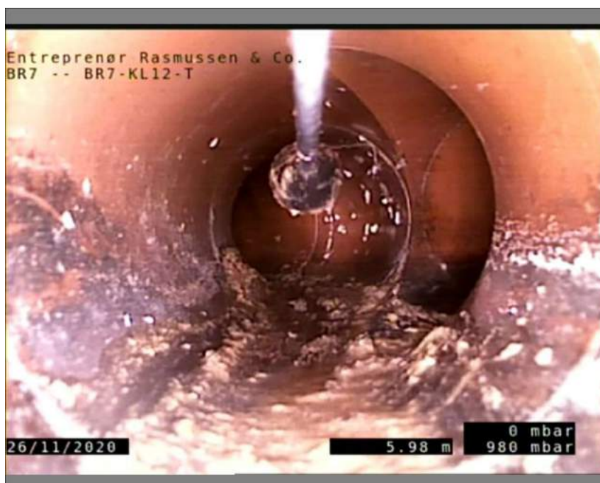
Foto: BR7-BR7-KL12-T-261120-5,98-5-A.JPG 5,98m, Grenrør Klasse 0, urref 3
