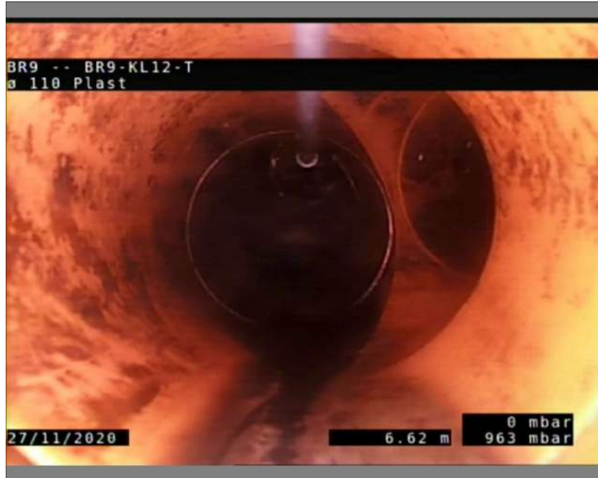
Foto: BR9-BR9-KL12-T-271120-6,62-5-A.JPG 6,62m, Grenrør Klasse 0, urref 3
